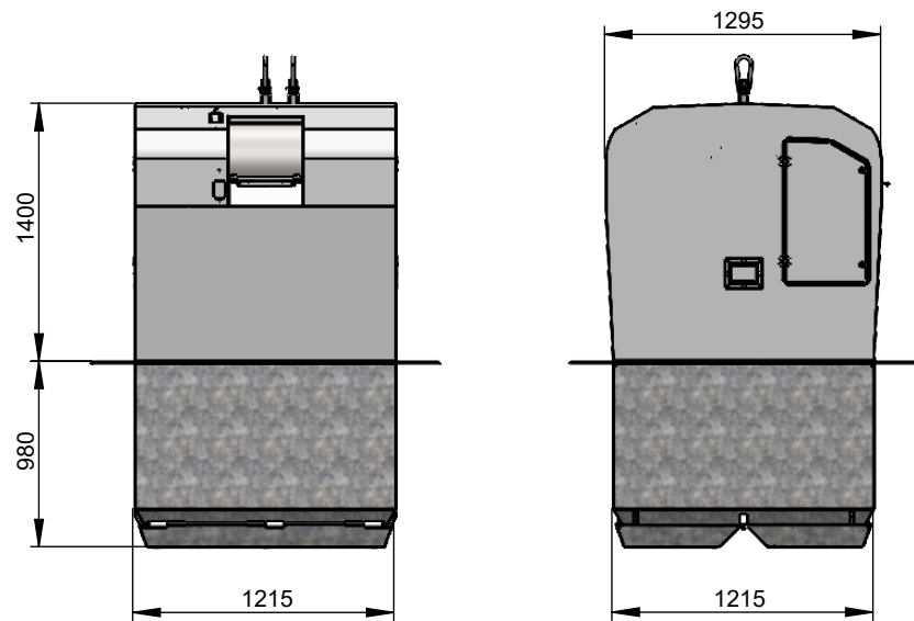
Volume 3m 3
